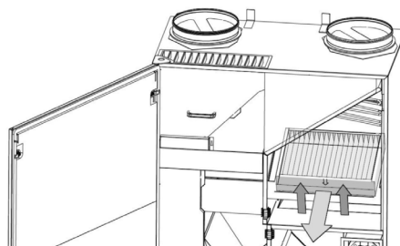
Binnenfilter (toevoerfilter)
