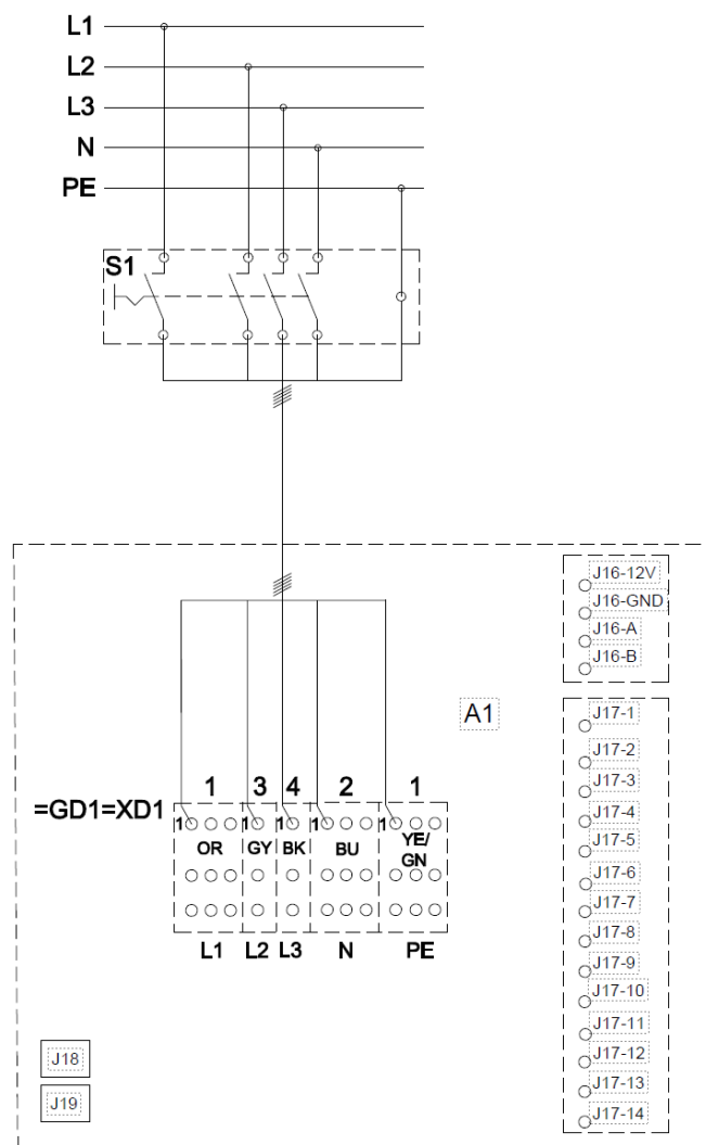
Afbeelding 8: Regelkast, standaardconfiguratie
