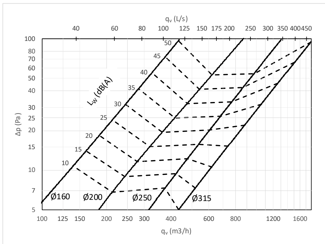
Afbeelding 1: Luchtvolumedebiet q_v [l/s]; [m³/h], drukval \Delta p [Pa] en geluidsdruk niveau LWA [dB(A)] worden in de grafiek weergegeven.
