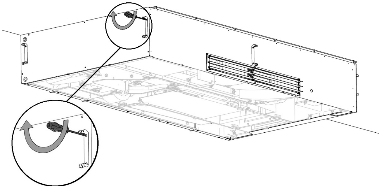
Afbeelding 25: Paneelbeugels monteren - 1
