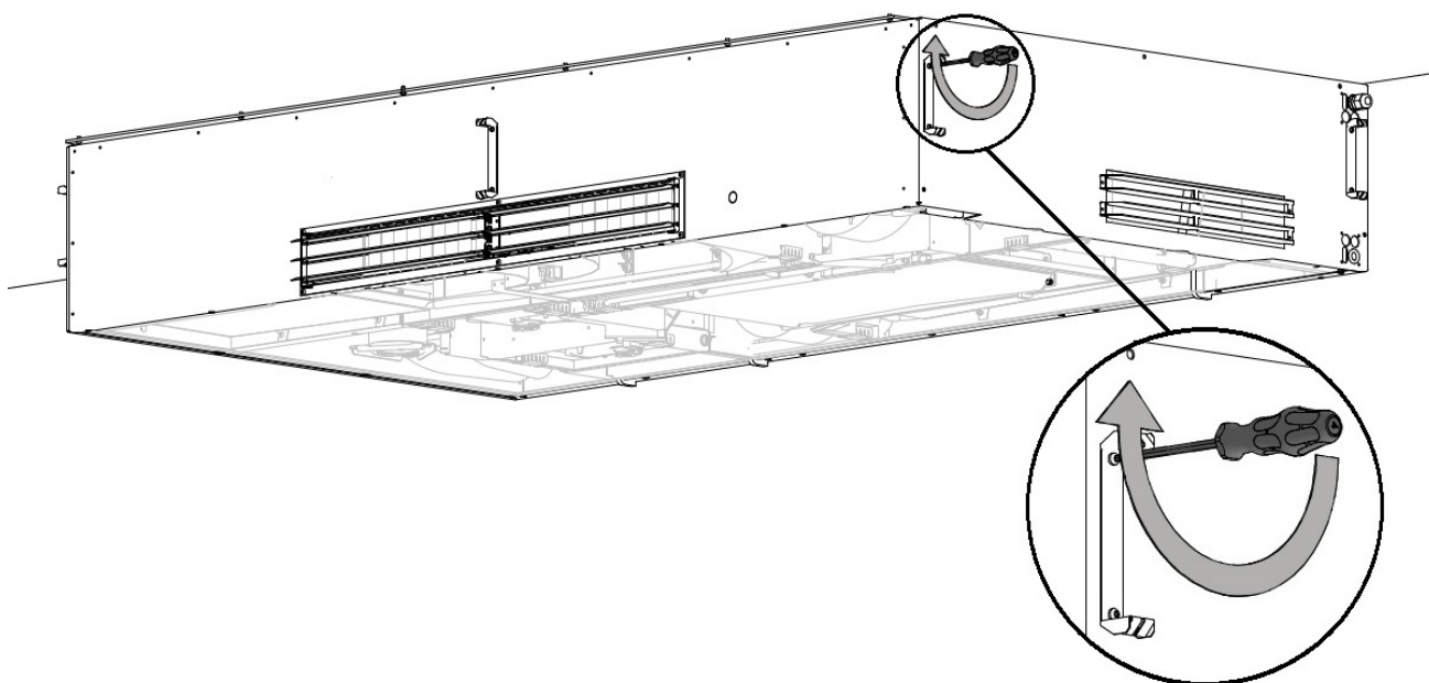
Afbeelding 26: Paneelbeugels monteren - 2
