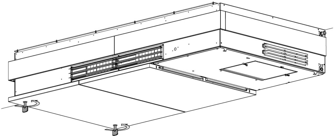
Afbeelding 55: De linker servicedeur vergrendelen
