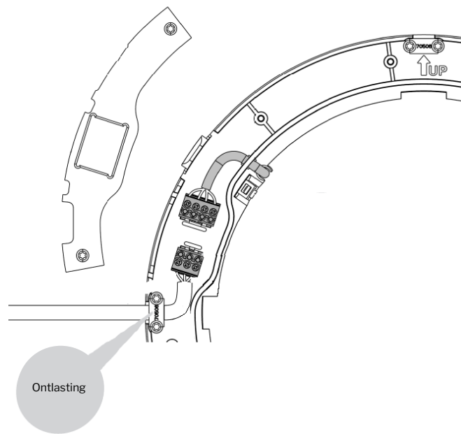
Afb. 39 - Kabelingang van links met ontlasting in klemmenstrook 3
