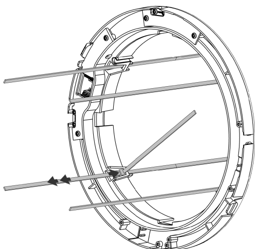
Afb. 22 - Kabelbinder wordt naar beneden geduwd
