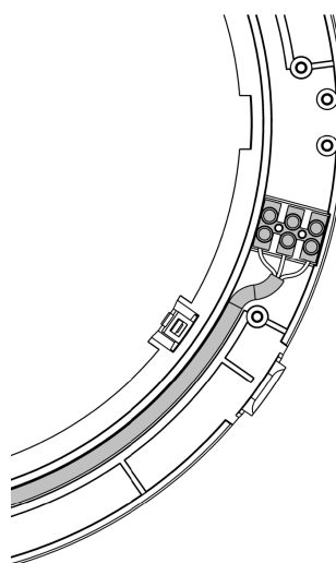
Afb. 34 - Interne kabel gemonteerd op klemmenstrook 2
