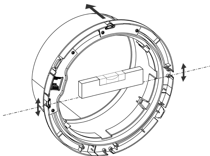
Afb. 19 - Aanbrengen van de binnenwandbekleding
